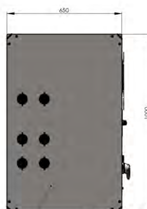
VUE DESSUS
